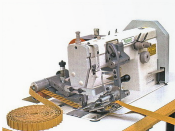
Mašina za šivanje VP 380 SGH 14CAM
